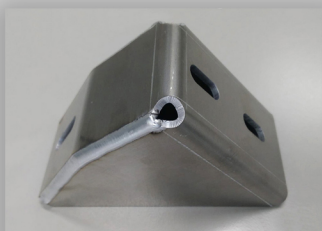
Staffe saldate
